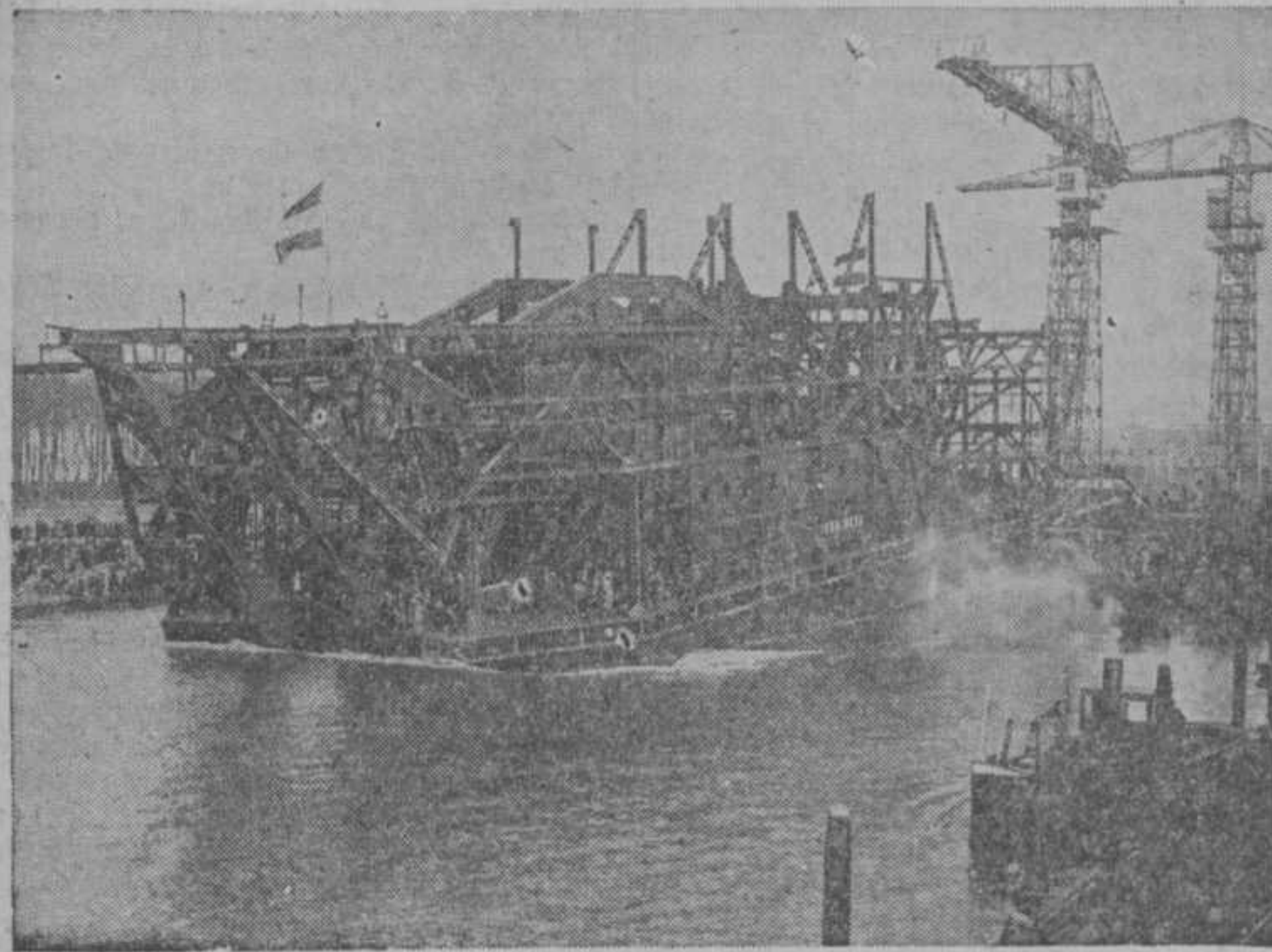
Zaterdagmiddag, 26 Febr. j.l., is de „Karimata“, 's werelds grootste tinbagger-molen, bestemd voor de Billiton Maatschappij, te water gelaten. Met de vlag fier in top glijdt het ijzeren gevaarte, dat naar Indië zal worden gesleept, doch eerst nog naar het goud van de „Lutine“ zal baggeren, het water in.
