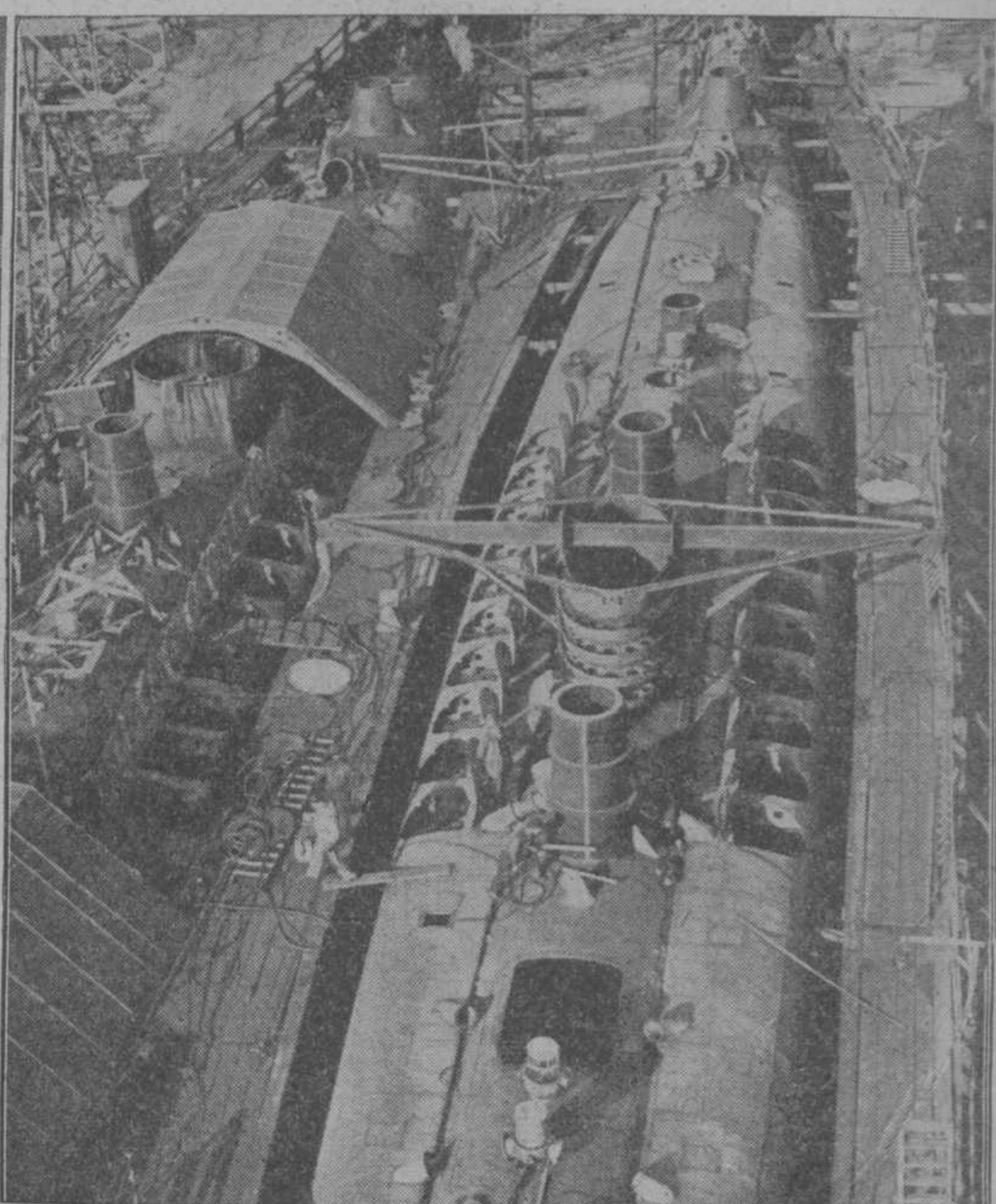
Onze grootste onderzeeërs. — De K. 19 en K. 20, de grootste onderzeeërs, tegelijk mijnenleggers, olt voor de Koninklijke marine gebouwd, liggen vlak naast elkaar op de Wilton-Fijnschroef te Schiedam. Zij zijn thans zoover gereed, dat de commando-torens geplaatst kunnen worden. — Links: de K. 20, gedeeltelijk onder de overkapping. Rechts: de K. 19, waarin duidelijk de „mijnenbuis” (met opgeklapt deksel) te zien zijn.
